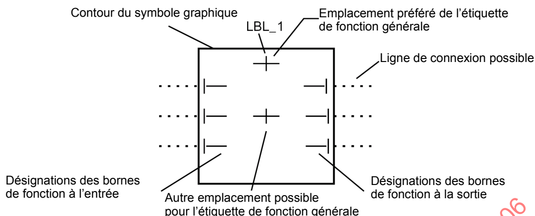
Figure 12 – Etiquettes générales dans les symboles graphiques et leur alignement
