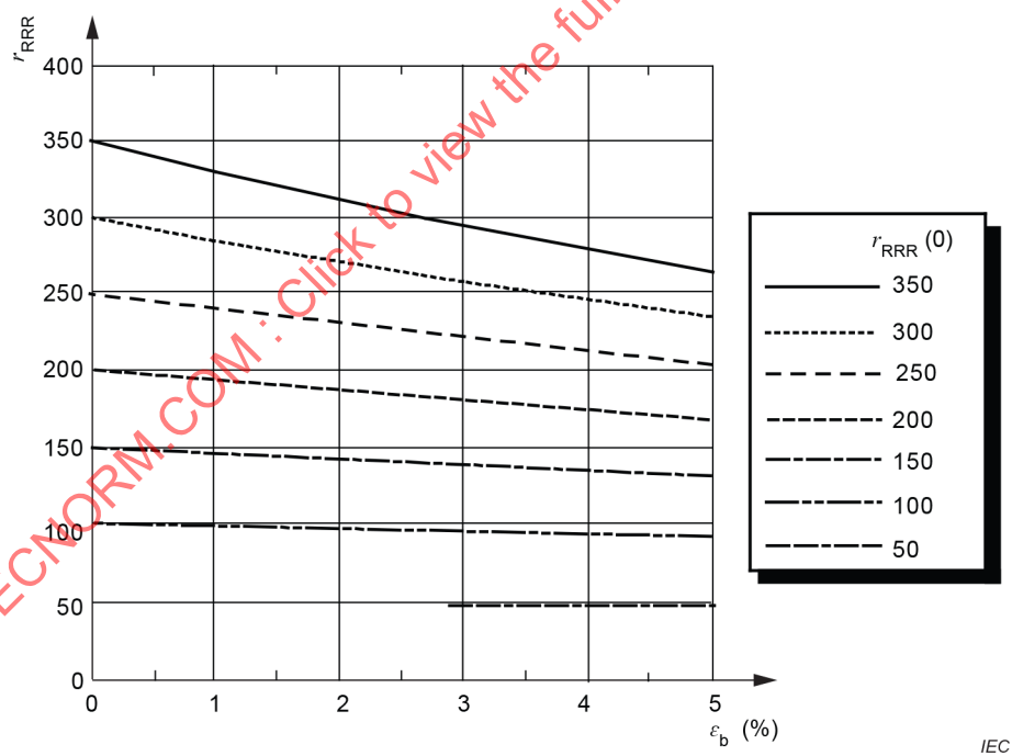
Figure A.5 – Dépendance de la valeur du RRR vis-à-vis de la flexion pour des fils de cuivre rectangulaires
