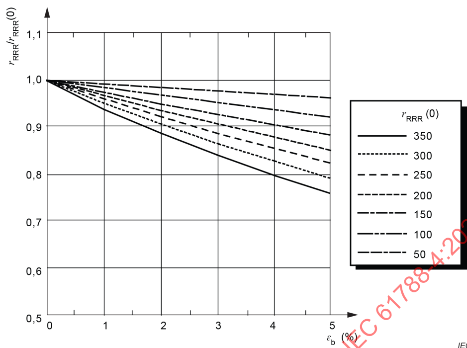
Figure A.6 – Dépendance de la valeur normalisée du RRR vis-à-vis de la flexion pour des fils de cuivre rectangulaires
