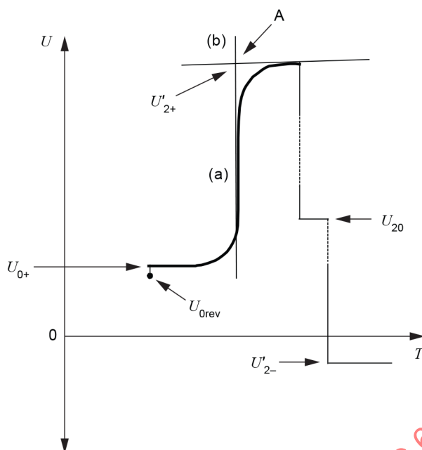
Figure A.1 – Définition des tensions
