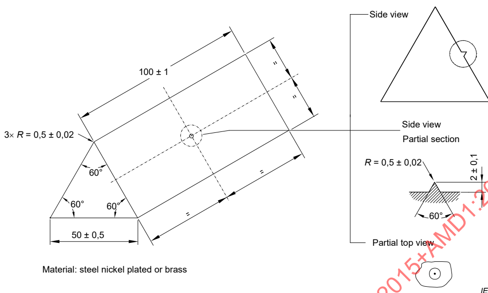
a) Mandrel
