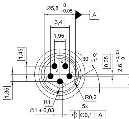
Figure 19 – Vue de face du contact mâle – Codage B
