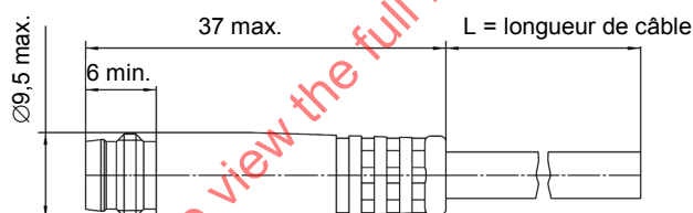
Figure 7 – Fiche non démontable, contacts mâles, version à sortie droite, à encliquetage
