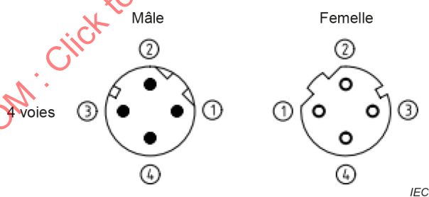
Figure 37 – Position des contacts détrompage D, vue de face
