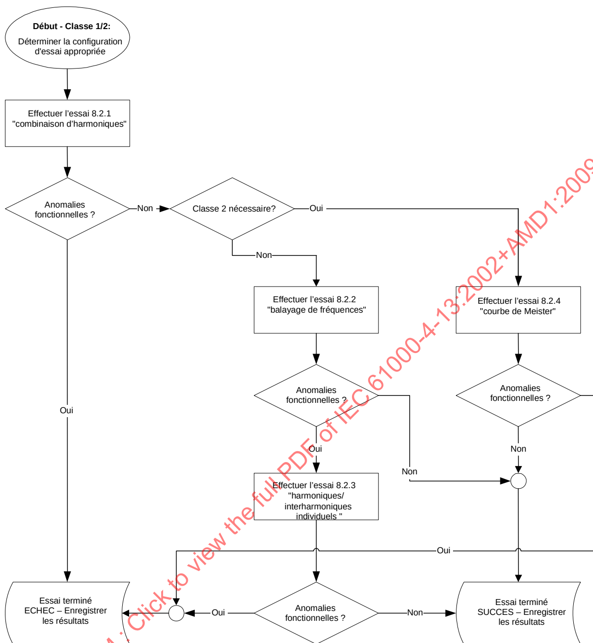
Figure 1a – Synoptique d'essai pour la classe 1 et pour la classe 2
