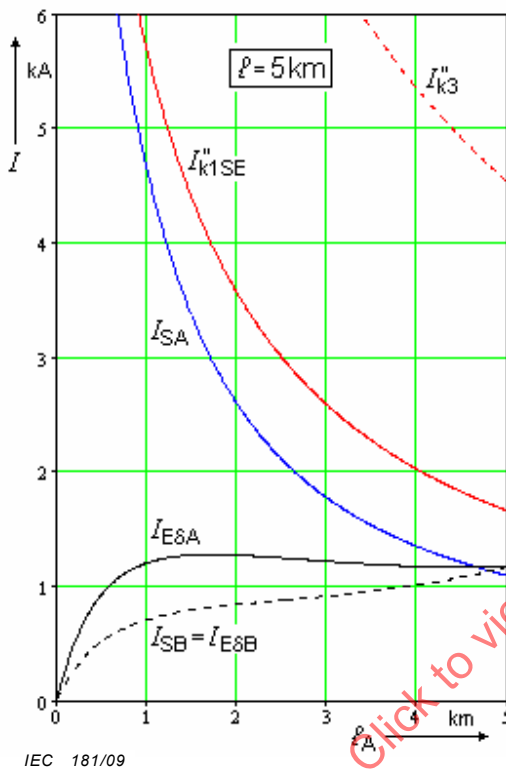
a) Longueur de câble \ell = 5 km
