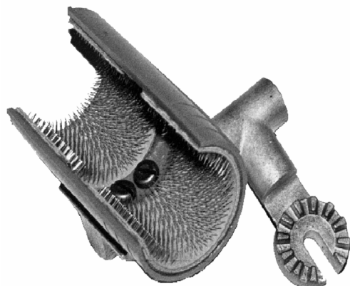
Semi-tubulaire - Semi-tubular
