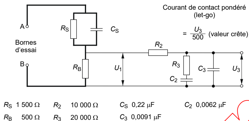
Figure G.3 – Réseau de mesure, courant de contact pondéré pour "let-go" (pour les luminaires portatifs de classe I)
