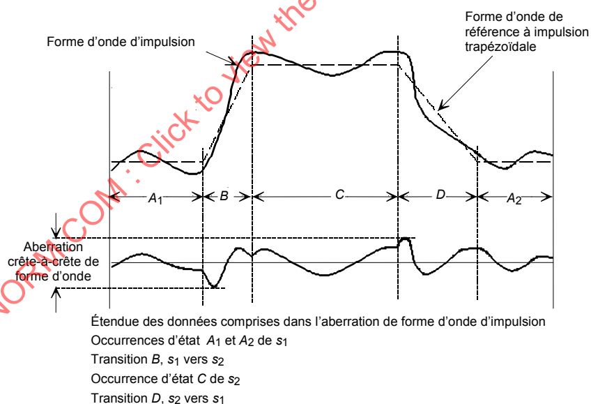
Figure 9 – Calcul de l'aberration de forme d'onde
