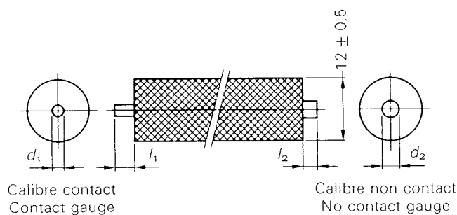
Calibre pour les prises mobiles 0,2 A et 2,5 A Gauge for 0,2 A and 2,5 A connectors
