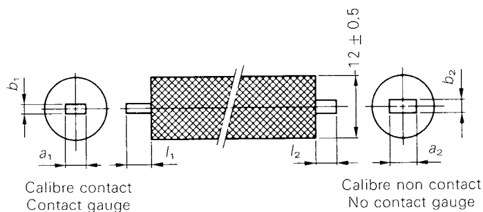
Calibre pour les prises mobiles 6 A, 10 A et 16 A Gauge for 6 A, 10 A and 16 A connectors
