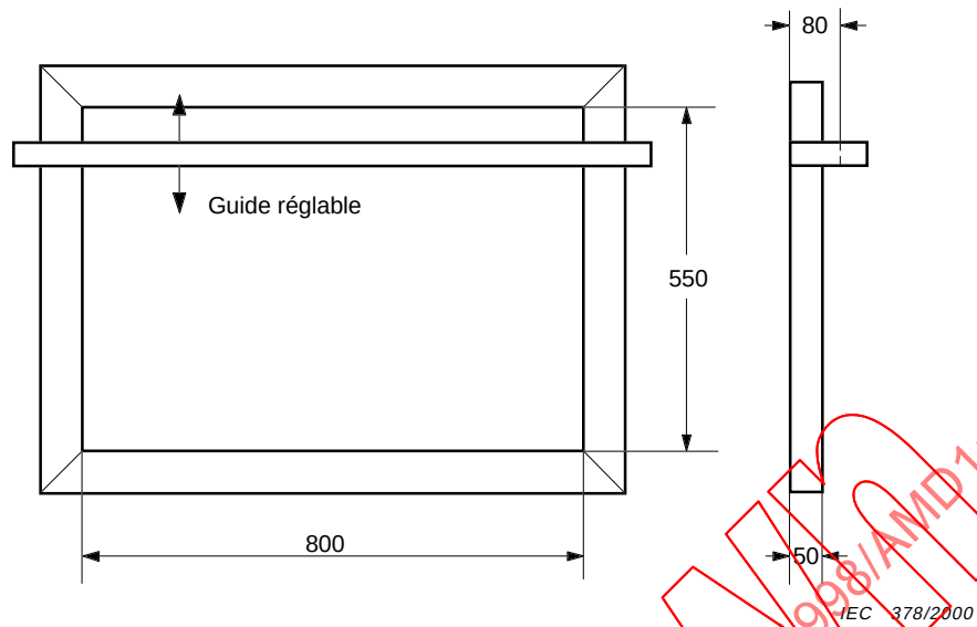
Figure 10B – Cadre pour coussin d'essai
