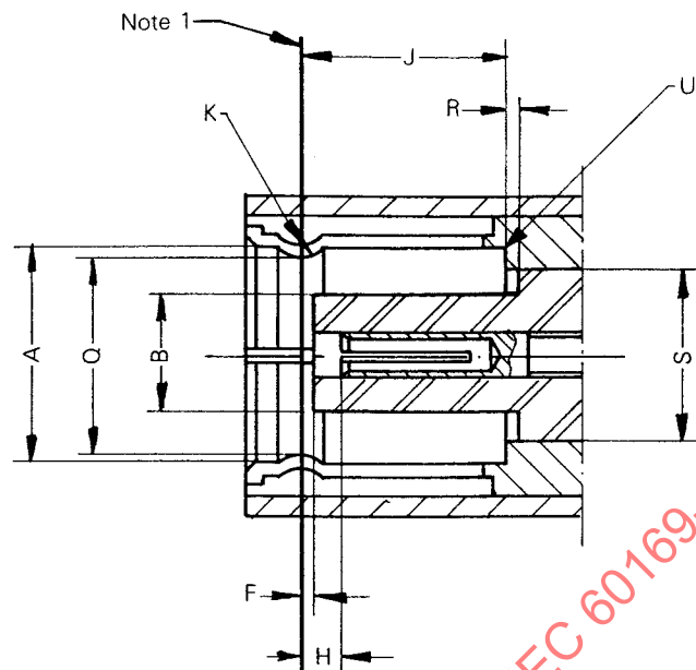
FIG. 6A. — Dimensions du connecteur (voir tableau). Dimensions of connector (see table).
