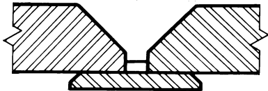
(d) Split Nub Type Backing Ring
